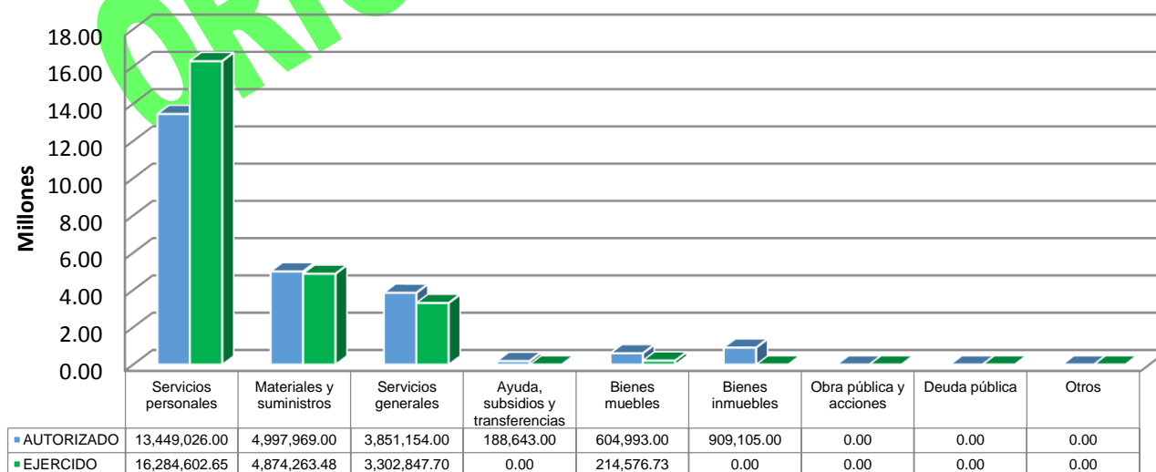
GRÁFICA 2 EGRESOS
